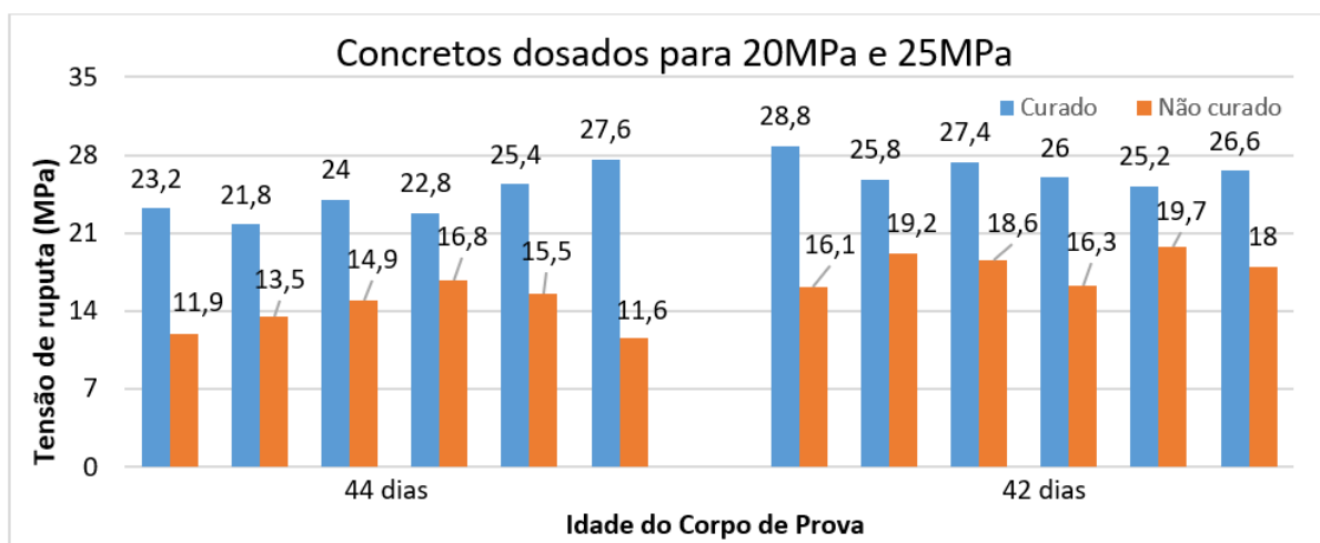
Figura 13: Resistência à compressão de corpos de prova curados e não curados
