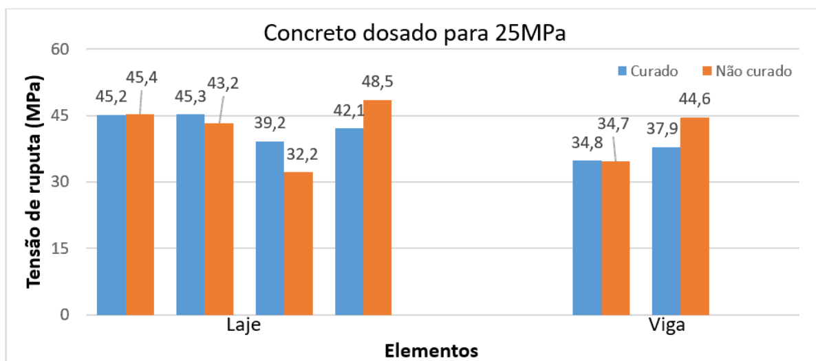
Figura 11: Resistência à compressão de concretos curado e não curado
