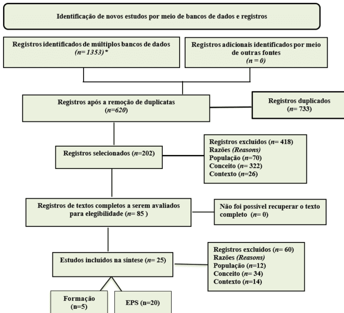
Figura 1: Flusso PRISMA-ScR
