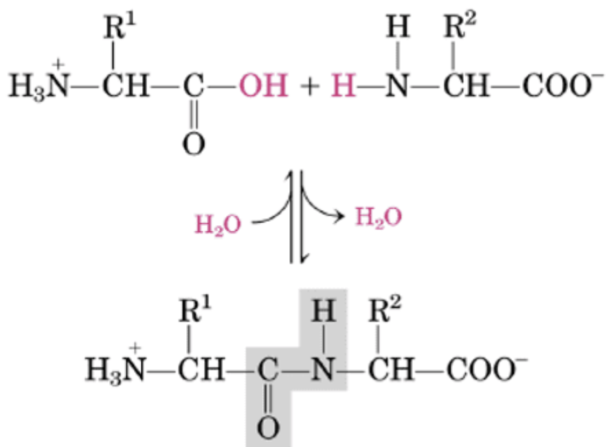
Figura 1. Ligação Peptídica.
