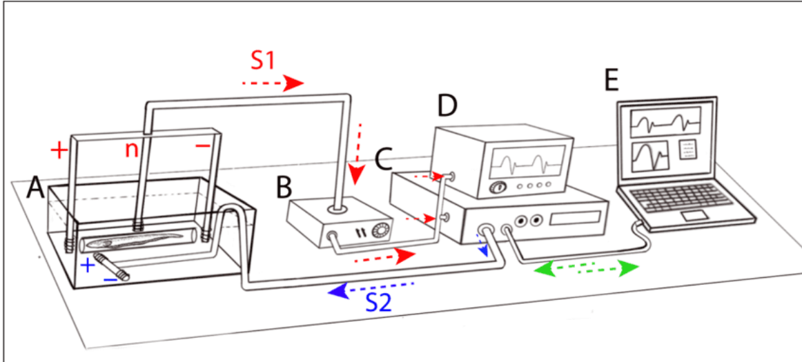
Figura 1: Representação esquemática de um arranjo experimental para experimentos comportamentais e de estimulação em peixes elétricos
